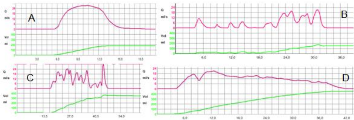
Figura 1. Formato das curvas de urofluxometria. A. Sino, B. Intermitente, C. Staccato, D. Platô
